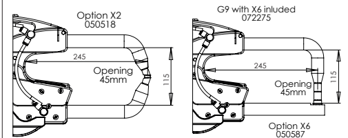
G9_X1 - 022881 - 8 bar / 550 daN G9_X6 - 072275 - 8 bar / 300 daN
