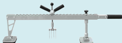
Barra de alineación doble acción ref. 053564
